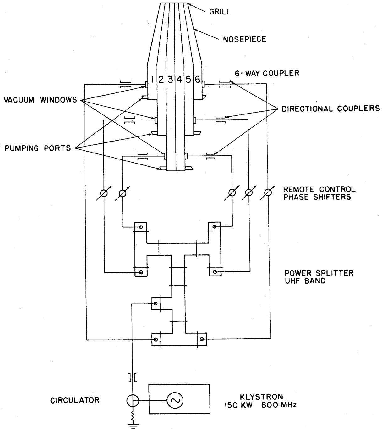
Fig. XX-4. RF system.
